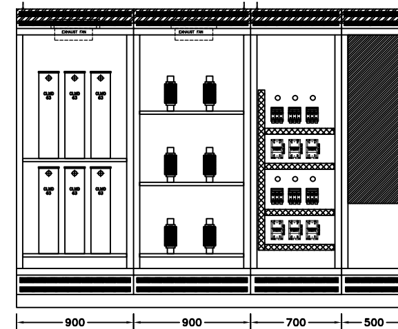
TAMPAK BELAKANG TERBUKA
