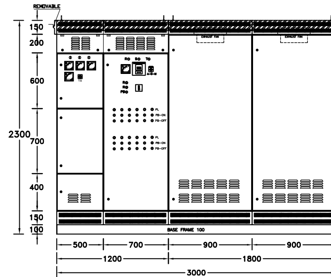
TAMPAK DEPAN TERTUTUP
