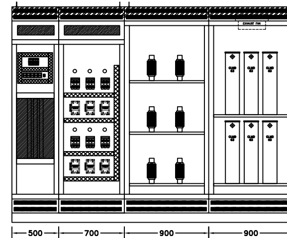
TAMPAK DEPAN TERBUKA
